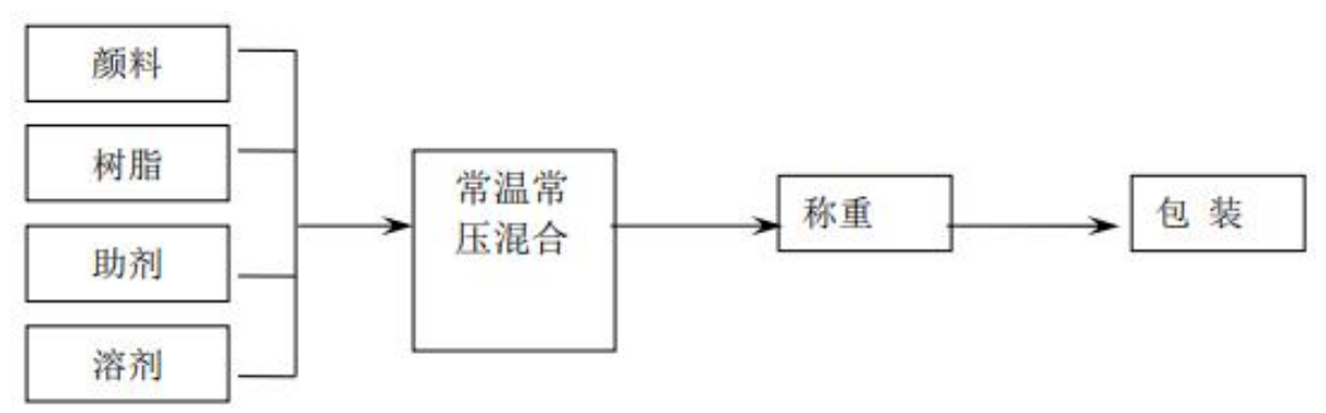
图 2.7-1 工业涂料工艺流程图
